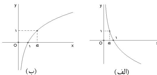
شکل ۲.۱۲: الف) تابع لگاریتمی با مبنی 0 < a < 1 ب) تابع لگاریتمی با مبنی 1 < a
