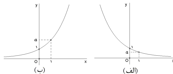
شکل ۲.۱۱: (الف) تابع نمایی با مبنی 0 < a < 1 (ب) تابع نمایی با مبنی a > 1
