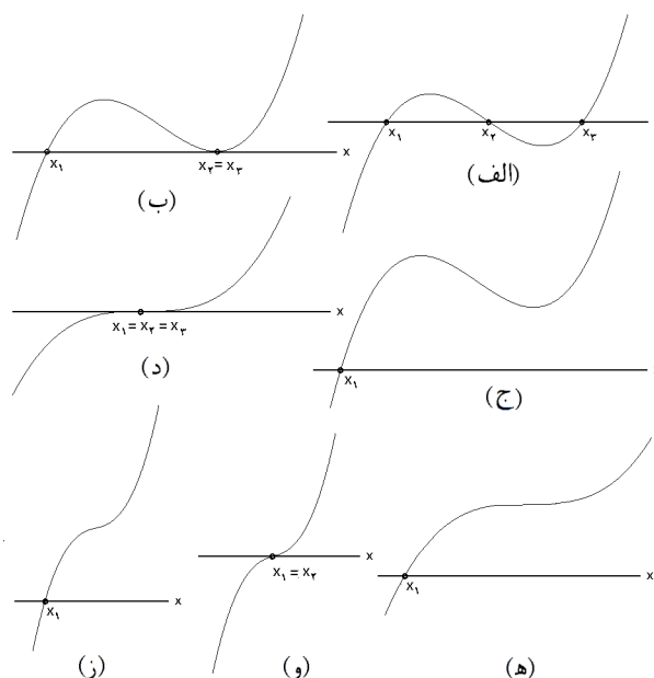
شکل ۲.۷: الف) تابع درجه سوم، \Delta > 0 و D < 0 ب) تابع درجه سوم، \Delta > 0 و D = 0 ج) تابع درجه سوم، \Delta > 0 و D > 0 د) تابع درجه سوم، \Delta = 0 و D > 0 ه) تابع درجه سوم، \Delta = 0 و D = 0 و) تابع درجه سوم، \Delta < 0 و D = 0 ز) تابع درجه سوم، \Delta < 0 و D > 0
