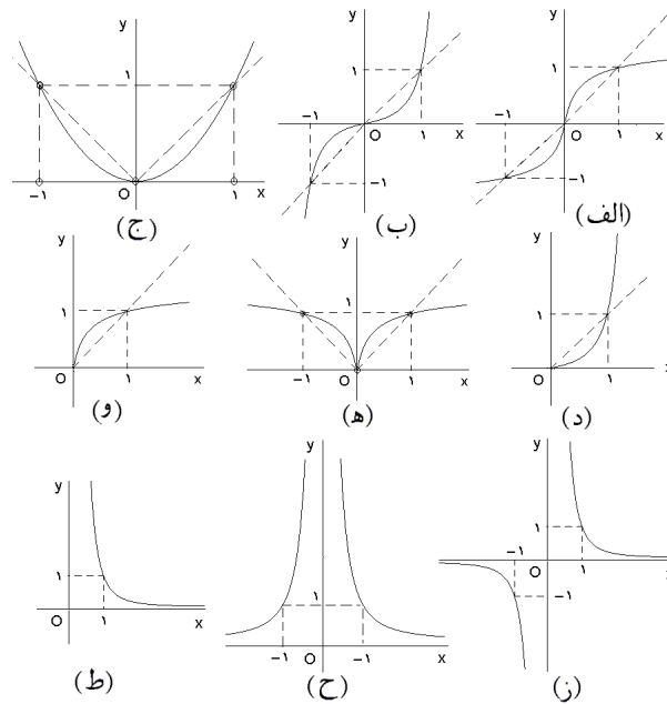
شکل ۲.۱۰: تابع y = x^{n/m} که (الف) m و n فرد و \frac{n}{m} > 1 (ب) m و n فرد و 0 < \frac{n}{m} < 1 (ج) n زوج، m فرد و \frac{n}{m} > 1 (د) m زوج، n فرد و \frac{n}{m} > 1 (ه) n زوج، m فرد و 0 < \frac{n}{m} < 1 (و) n زوج، m زوج و \frac{n}{m} > 1 (ز) n زوج، m زوج و 0 < \frac{n}{m} < 1 (ح) n فرد، m زوج و \frac{n}{m} > 1 (ط) n فرد، m زوج و 0 < \frac{n}{m} < 1 (ث) n فرد، m فرد و \frac{n}{m} > 1 (ج) n فرد، m فرد و 0 < \frac{n}{m} < 1
