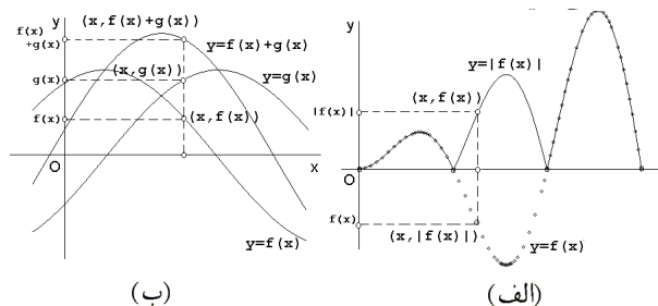
شکل ۲.۲۷: (الف) تابع y = |f(x)| (ب) تابع y = f(x) + g(x) با a < 0
